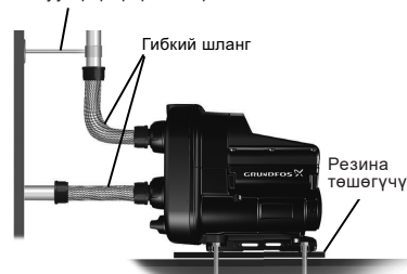
7-сүрөт. SCALA2 үчүн ызы-чууну азайтуу боюнча иш-чаралар
