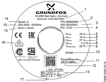
Նկար 3 Ֆիրմային վահանակի օրինակ
