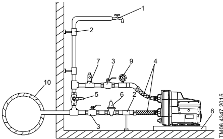
Նկար 8 Ջրմուղային խողովակաշարի ջրի ճնշման բարձրացում
