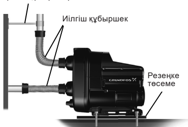
7-сур. SCALA2 шуын азайту шаралары
