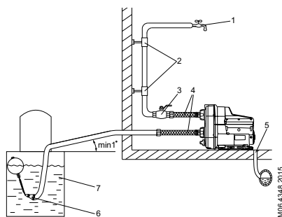
Рис. 10 Подача воды из резервуара
