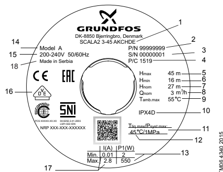
3-сур. Фирмалық тақтайша мысалы
