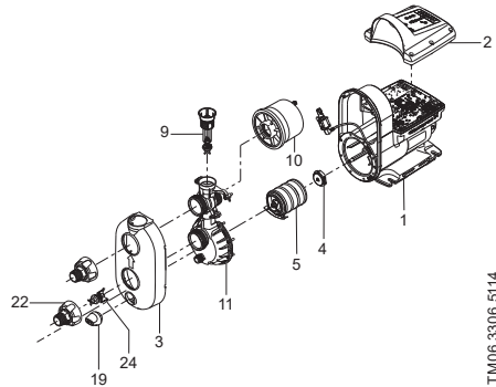
Նկար 2 SCALA2-ի կառուցվածք
