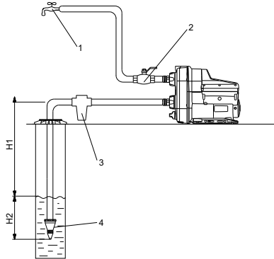
Նկար 9 Ջրի մատակարարումը ջրհորից/ հորանցքից
