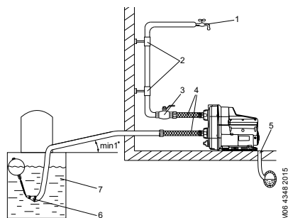
10-сур. Резервуардан су беру
