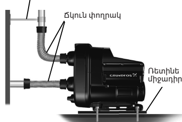
Նկար 7 SCALA2-ի աղմուկի նվազեցման համար միջոցառումներ
